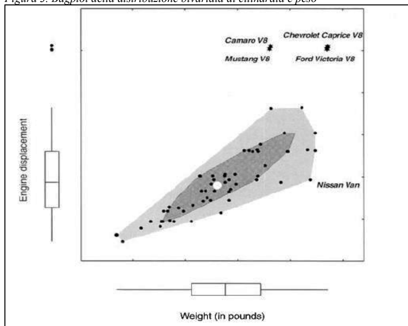
Figura 3. Bagplot della distribuzione bivariata di cilindrata e peso
